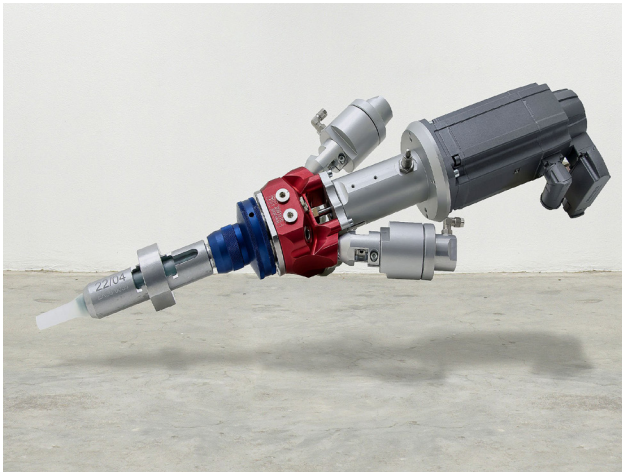
Zu den Stärken von TARTLER zählt die Entwicklung und Fertigung innovativer Mischköpfe für die Kunstharz-Verarbeitung. Im Bild ein LC 7/3 Rev.02 mit selbstschneidendem Mischeranschluss.
